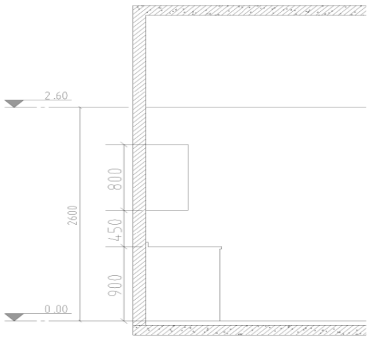
图 2-处置室治疗台剖面图
