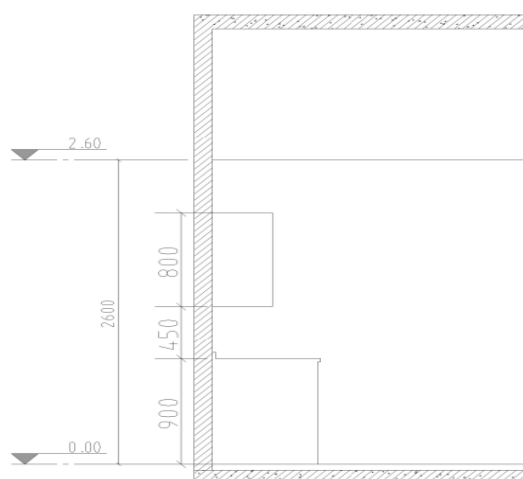
图 6-治疗室治疗台剖面图
